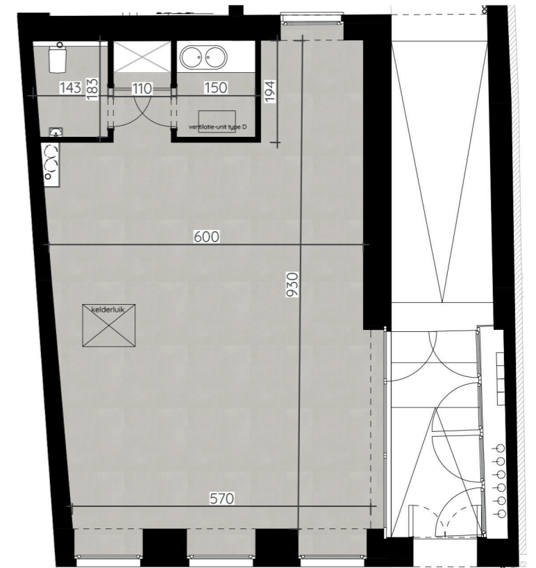
- grondplan 0 -
