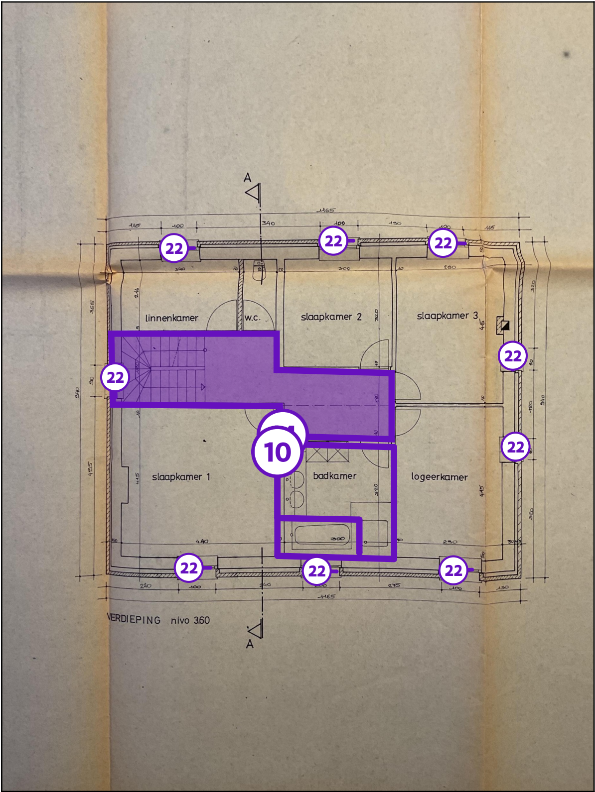
Legende van plan 1.6: Plan van de eerste verdieping
