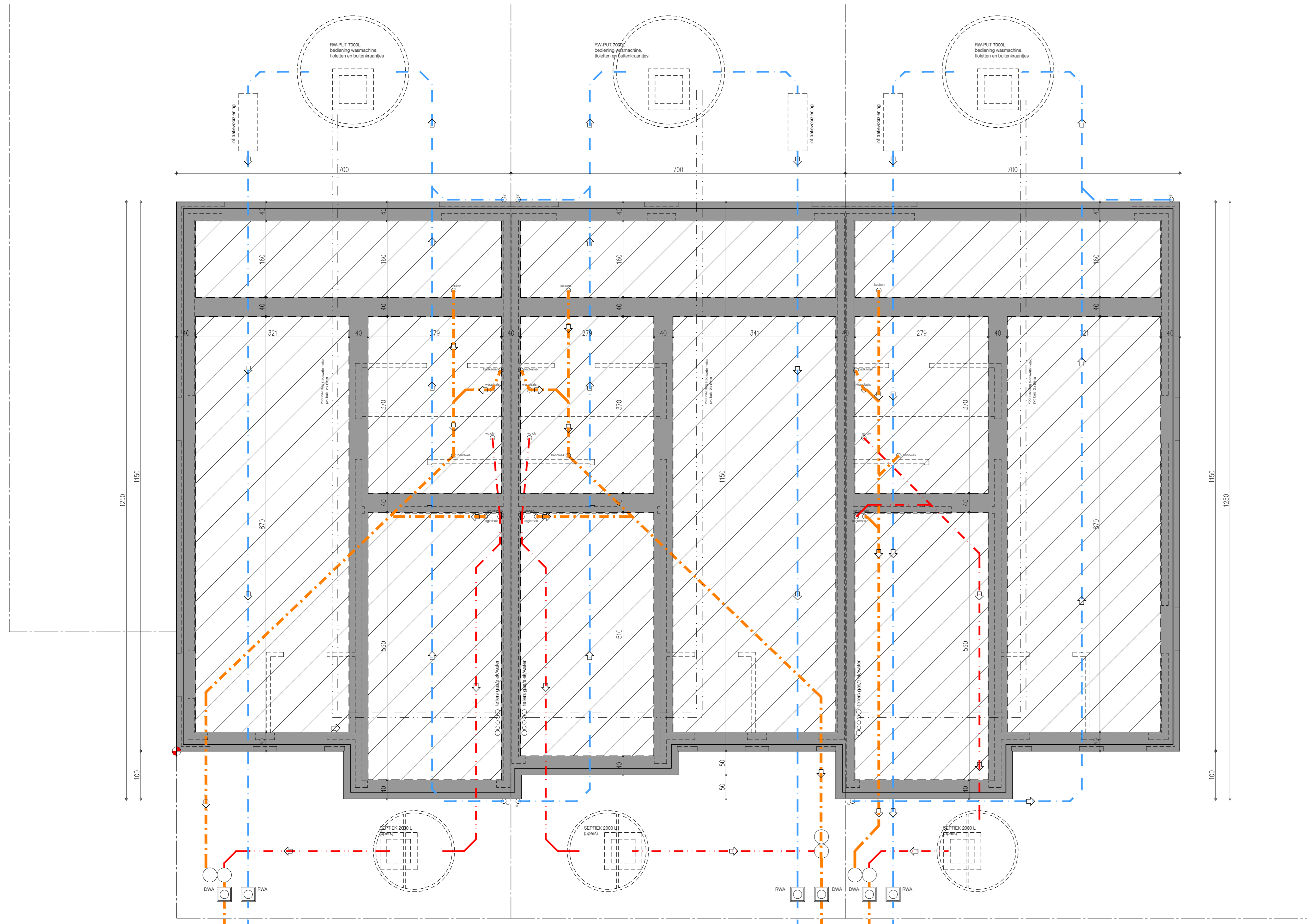
riolerings- en funderingsplan lot 6 riolerings- en funderingsplan lot 5 riolerings- en funderingsplan lot 4
