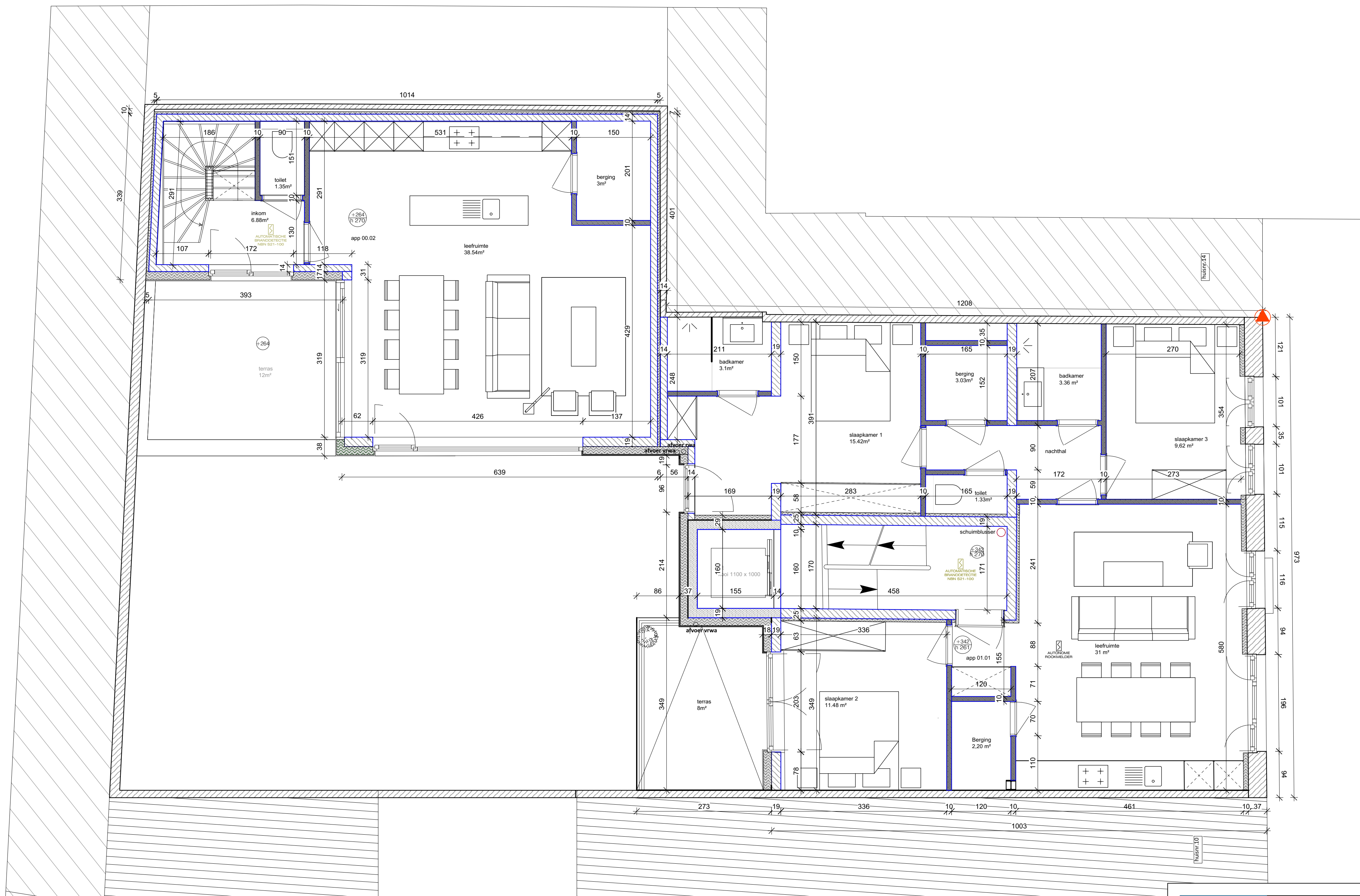
GRONDPLAN VERDIEP 1
