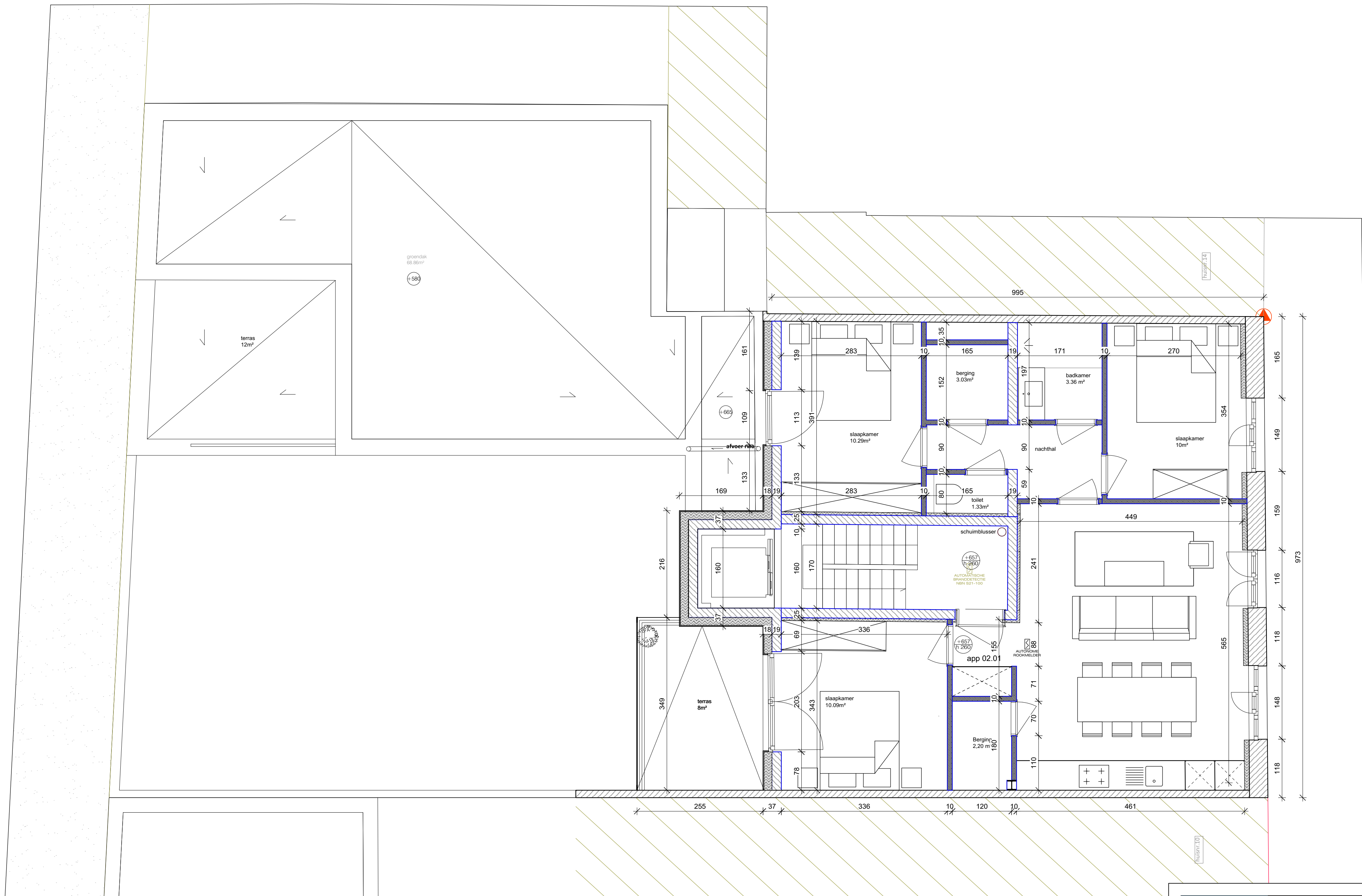
GRONDPLAN VERDIEP 2
