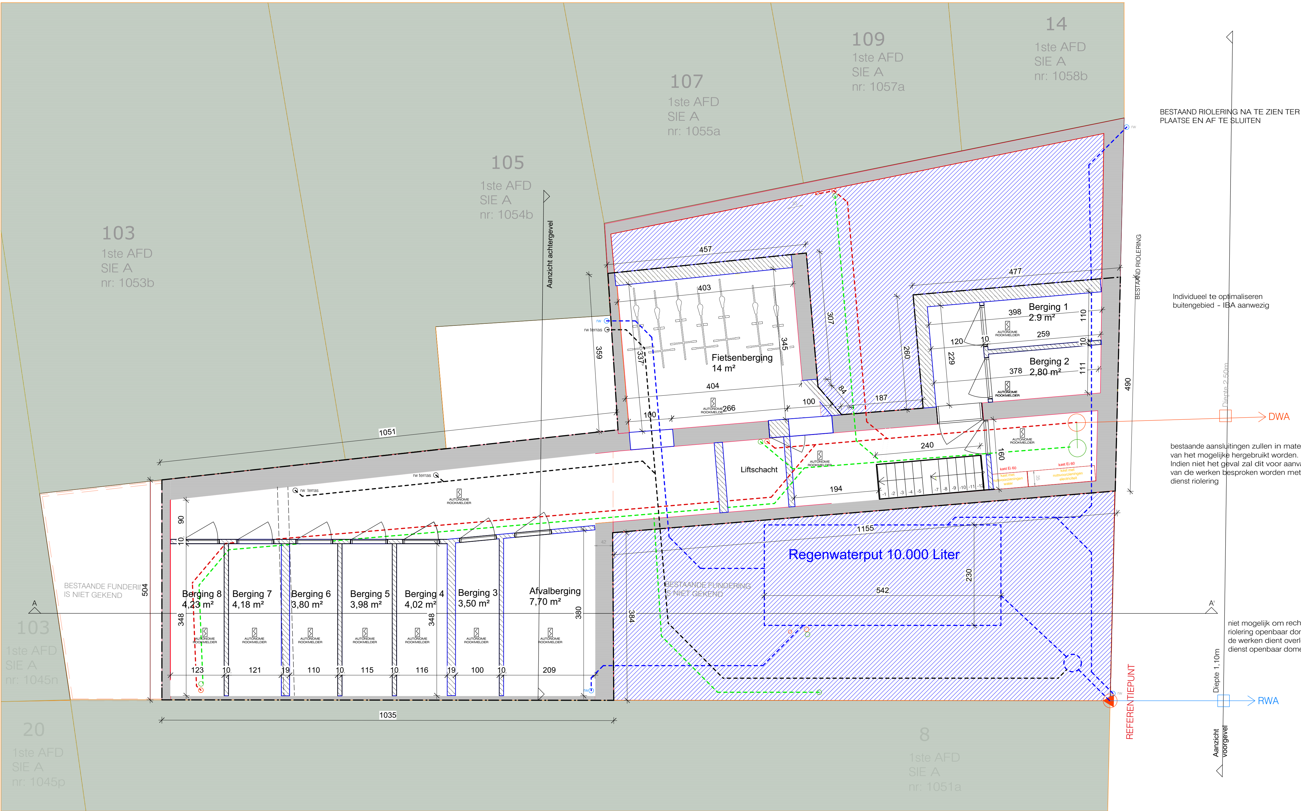
Grondplan kelder & rioleringen schaal 1/50
