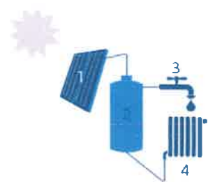
1 Zonnecollector | 2 Opslagvat zonnepaneel | 3 Sanitair warm water | 4 Afgeeft element voor ruimteverwarming (optioneel)
