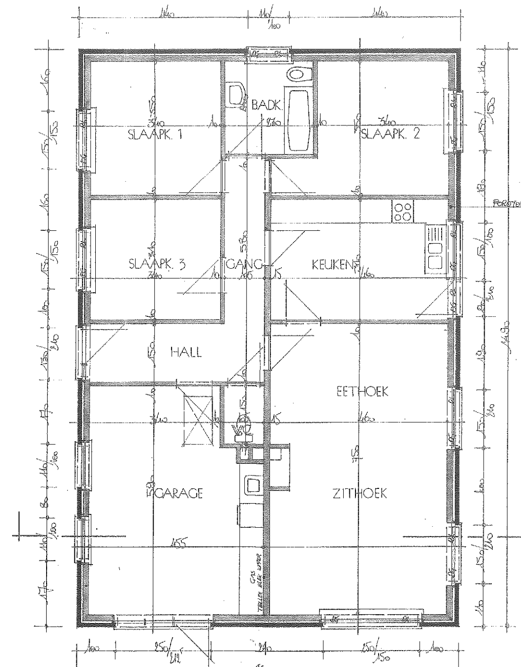
GELIJKVLOERS
