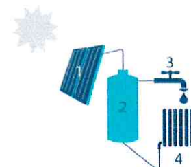
1 Zonnecollector | 2 Opslagvat zonneboiler | 3 Sanitair warm water | 4 Afgifteenheid voor ruimteverwarming (opulver)
