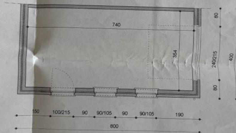
GRONDPLAN
