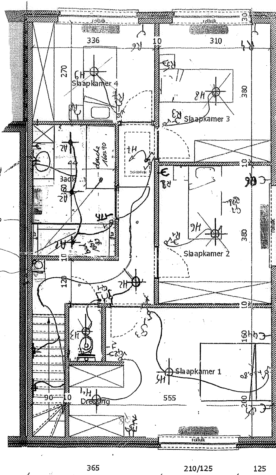
VERDIEPINGSPLAN
