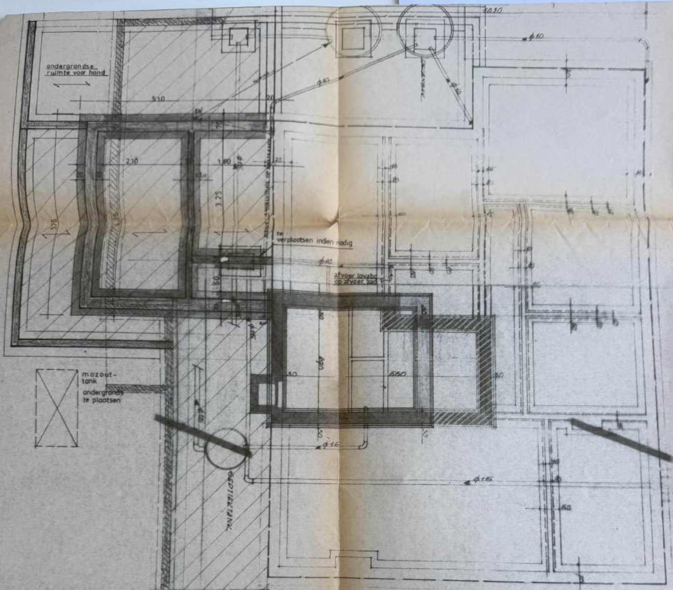
uitbreiding fundering-riolering
