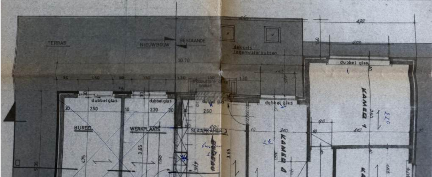
uitbreiding fundering-riolering
