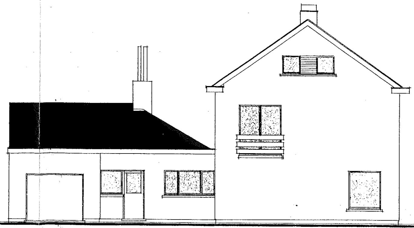
GEVEL. LINKS.
