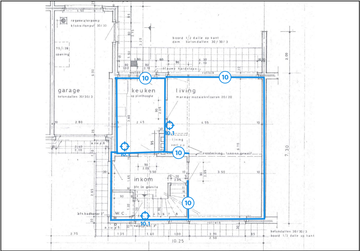
Legende van plan 1.10: Plan gelijkvloers
