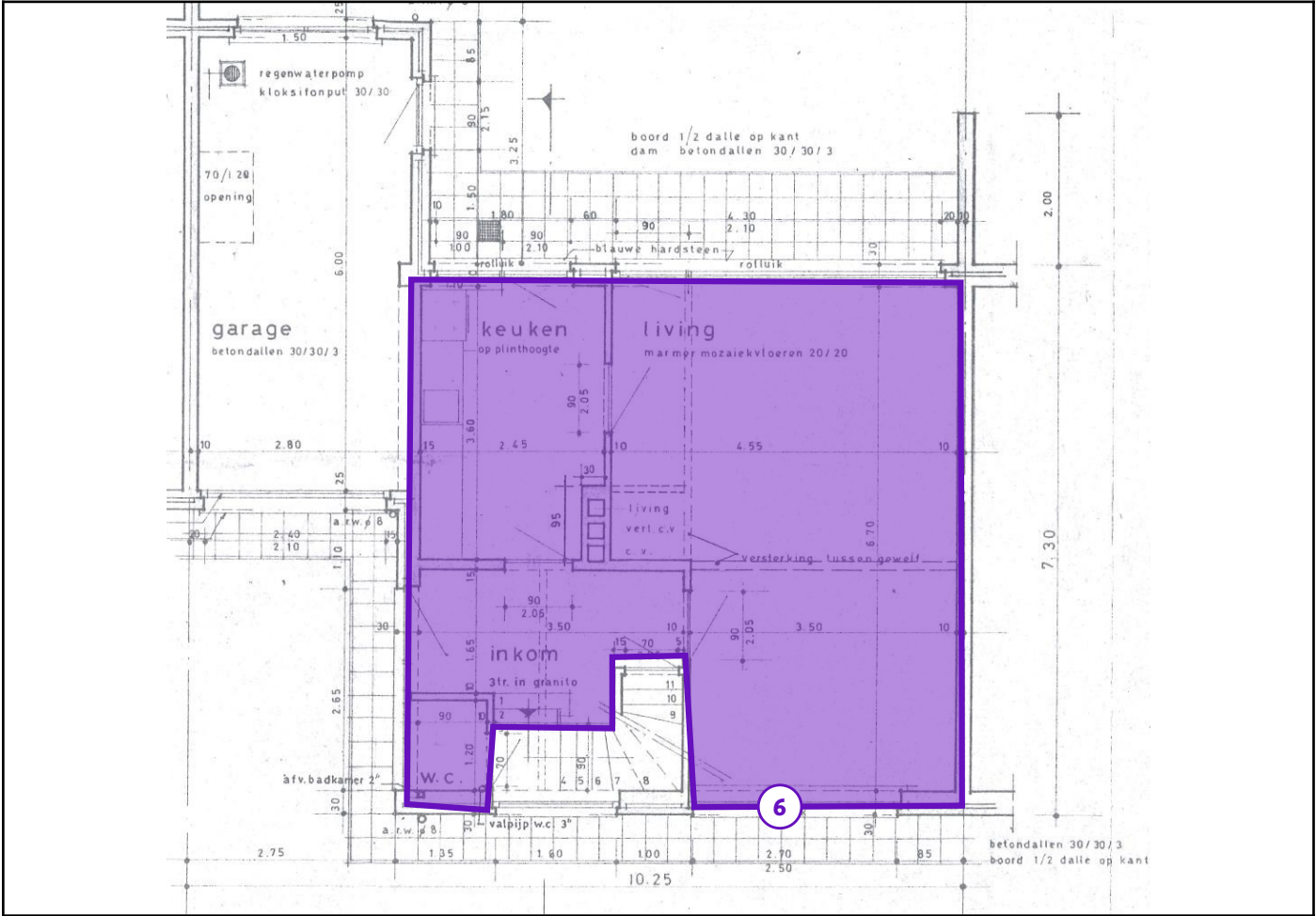
Legende van plan 1.5: Plan gelijkvloers
