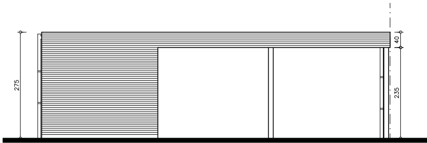
ZIJGEVEL LINKS
