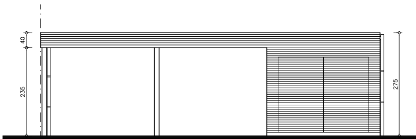
ZIJGEVEL RECHTS
