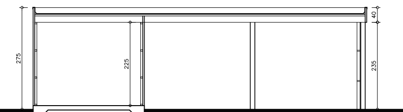
DOORSNEDE
