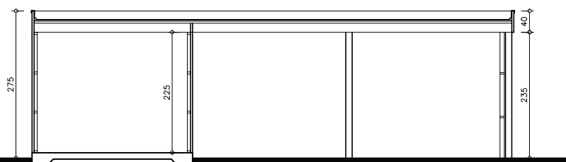
DOORSNEDE
