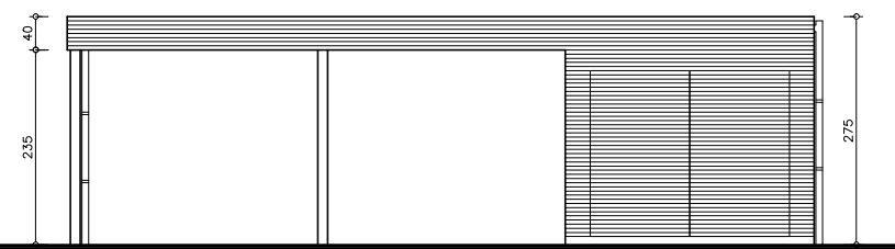
ZIJGEVEL RECHTS
