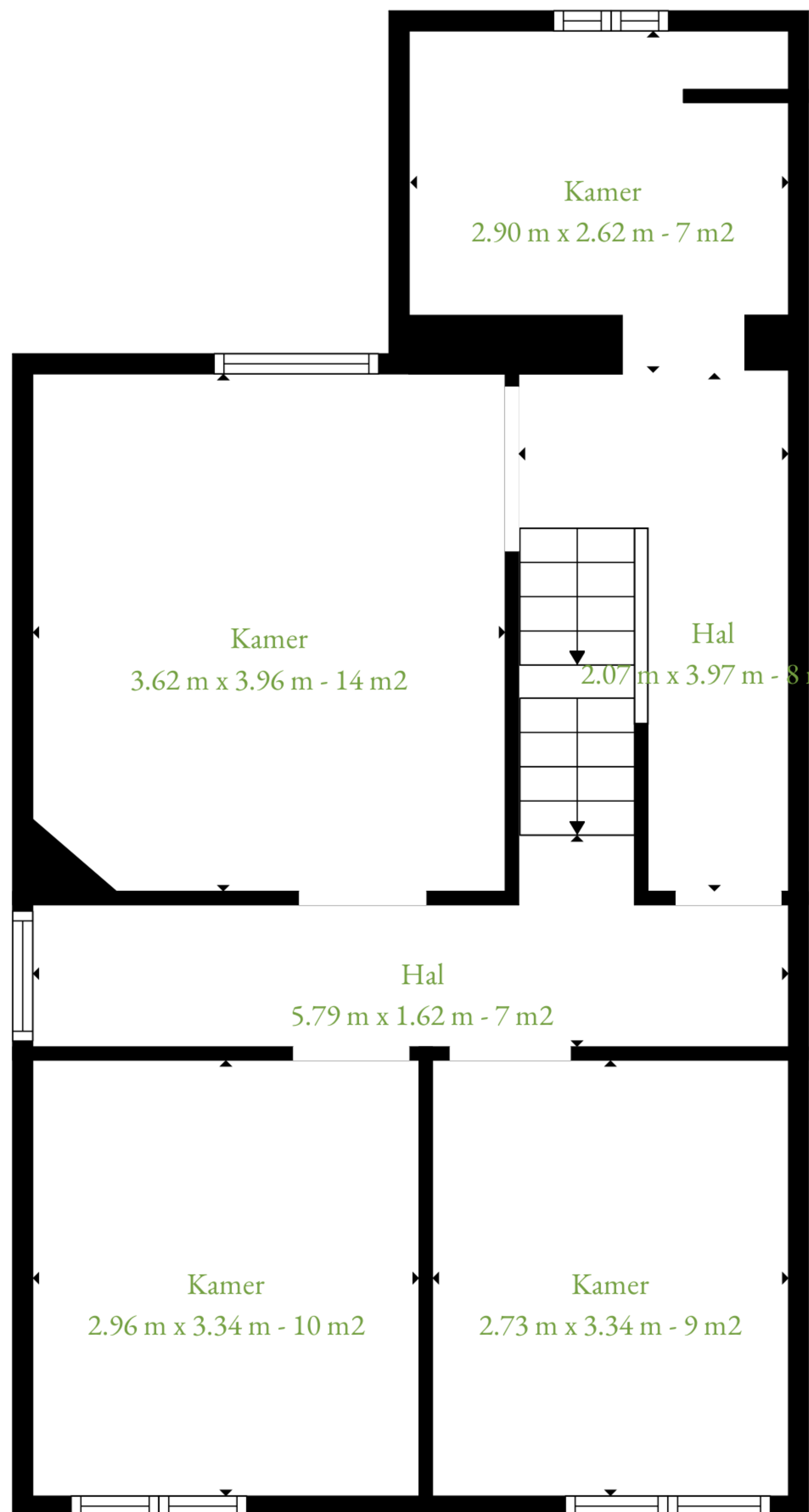
2. Verdieping
