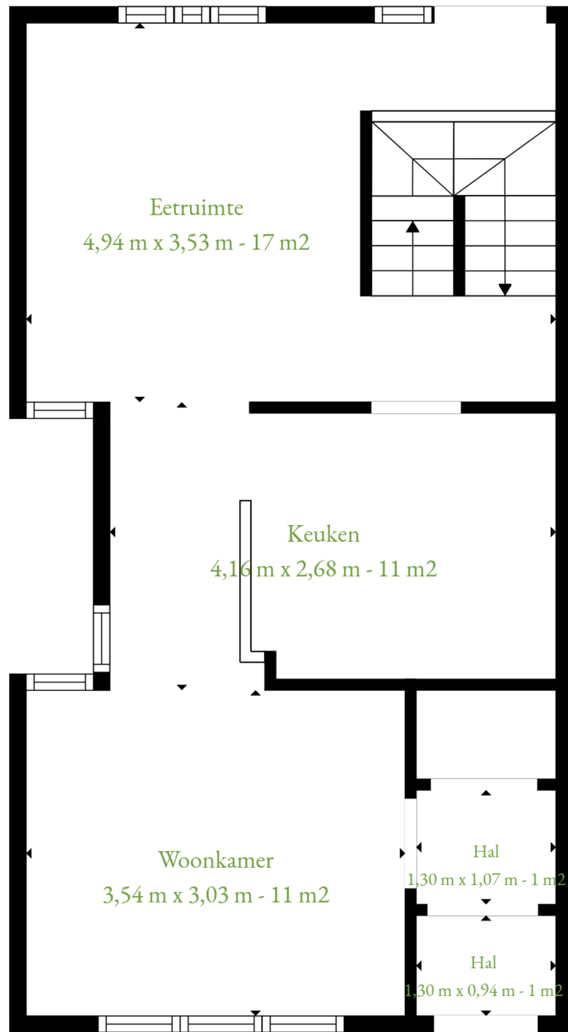
1e Verdieping
