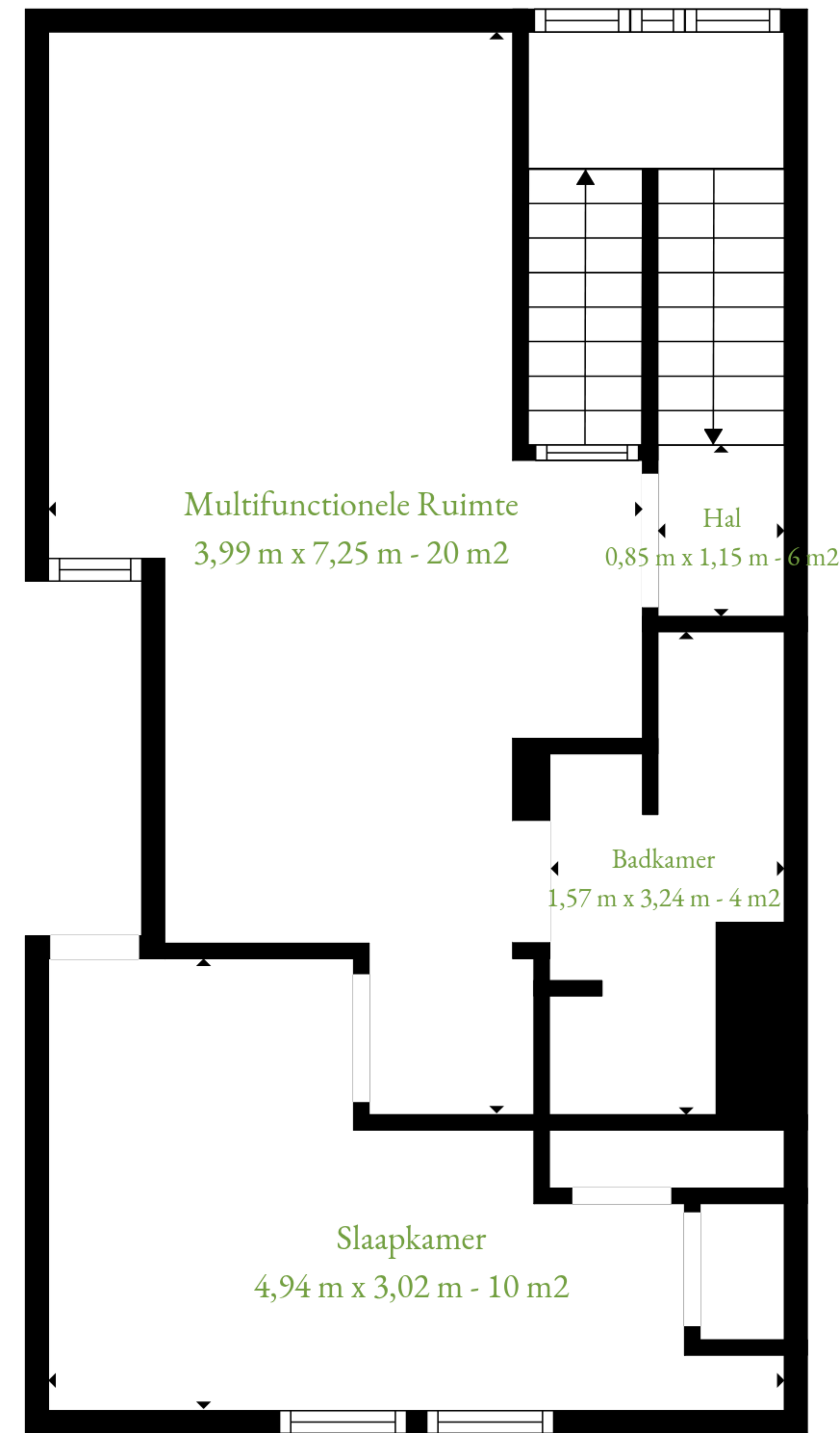
3e Verdieping
