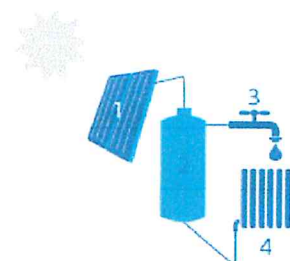
1 Zonnecollector | 2 Opslagvat zonneboiler | 3 Sanitair warm water | 4 Afgifteenheid voor ruimteverwarming (opfornsel)
