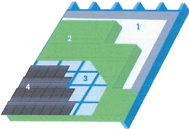
1. Dampschermb | 2. Isolatie | 3. Onderdak | 4. Dakbekleding
