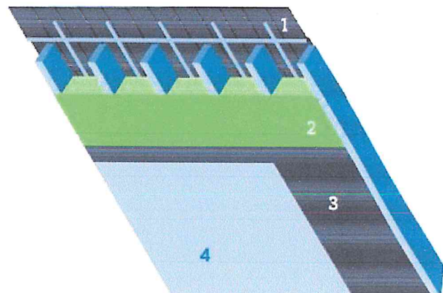
1. Onderdak | 2. Isolatie | 3. Dampschermb | 4. binnenafwerking
