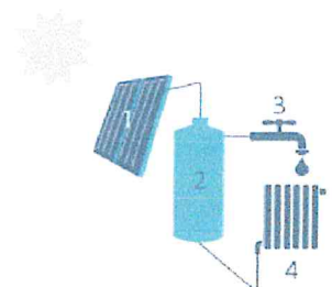
1 Zonnecollector | 2 Opslagvat zonneboiler | 3 Sanitair warm water | 4 Afgifteelement voor ruimteverwarming (op toestel)
