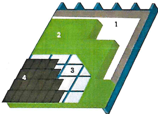
1. Dampscherm | 2. Isolatie | 3. Onderdak | 4. Dakbedekking
