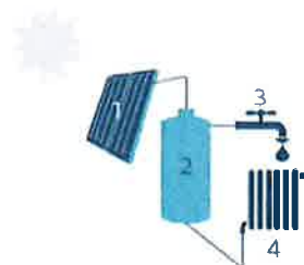
1 Zonnecollector | 2. Opslagvat warmwater | 3 Sanitair warm water | 4 Afschermend voor ruimteverwarming (optioneel)
