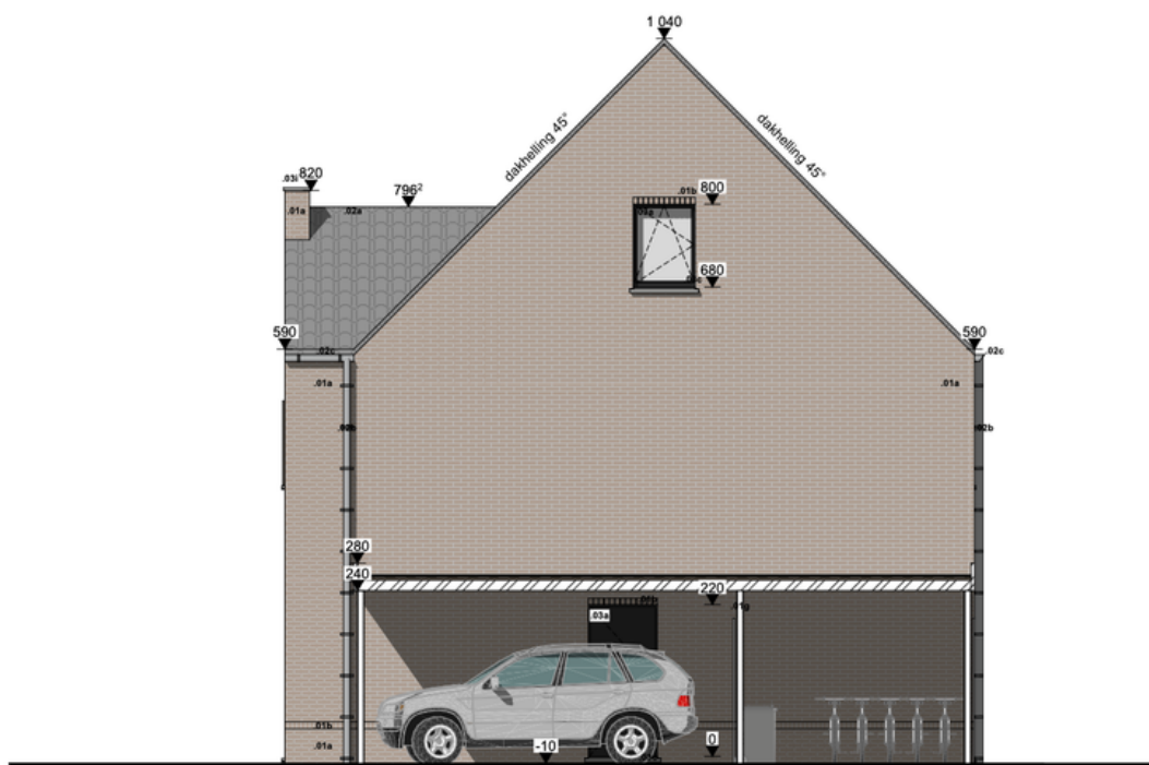
Rechtergevel
