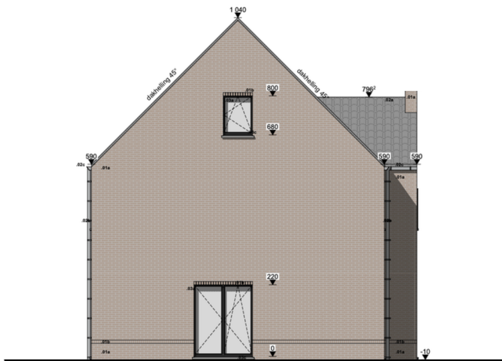
Linkergevel
