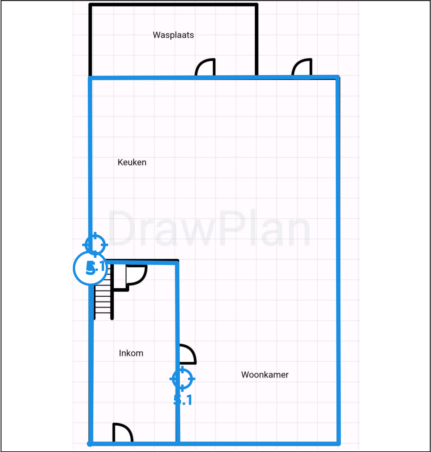
Legende van plan 1.3: Gelijkvloers : pleisterwerk wanden
