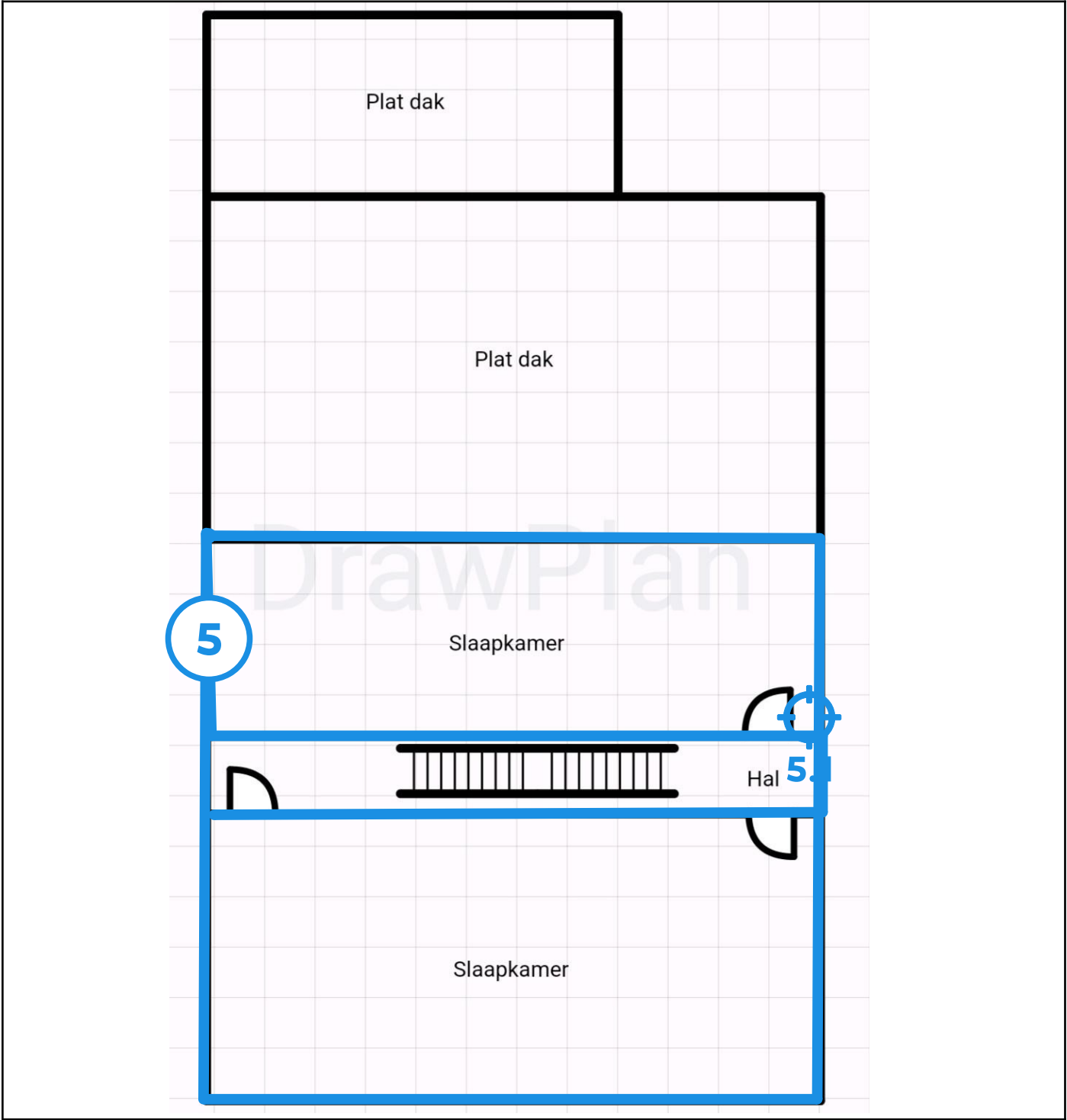
Legende van plan 1.11: Verdiep +2 : pleisterwerk wanden
