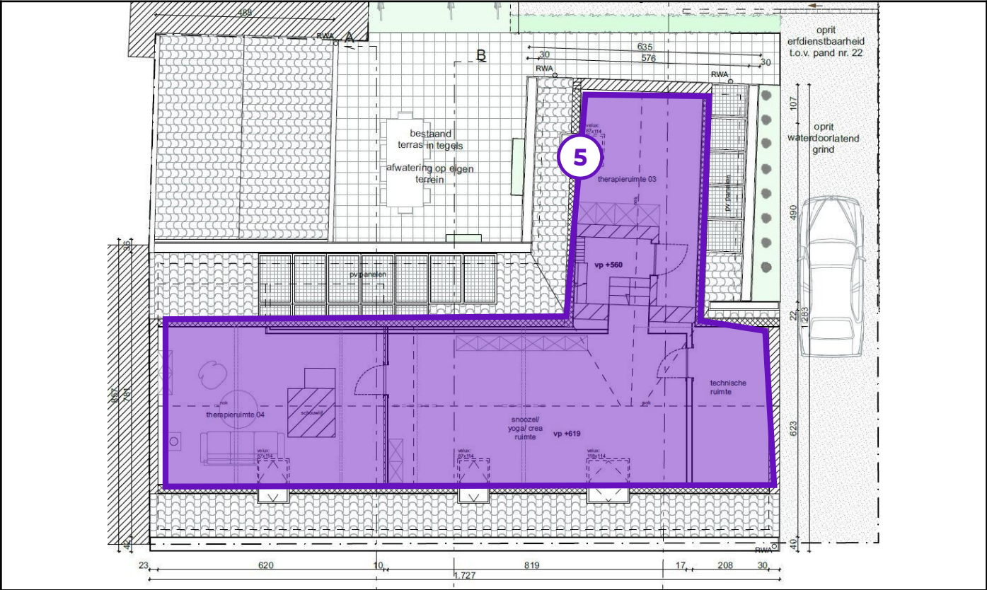
Legende van plan 1.5: Plan 2de verdieping
