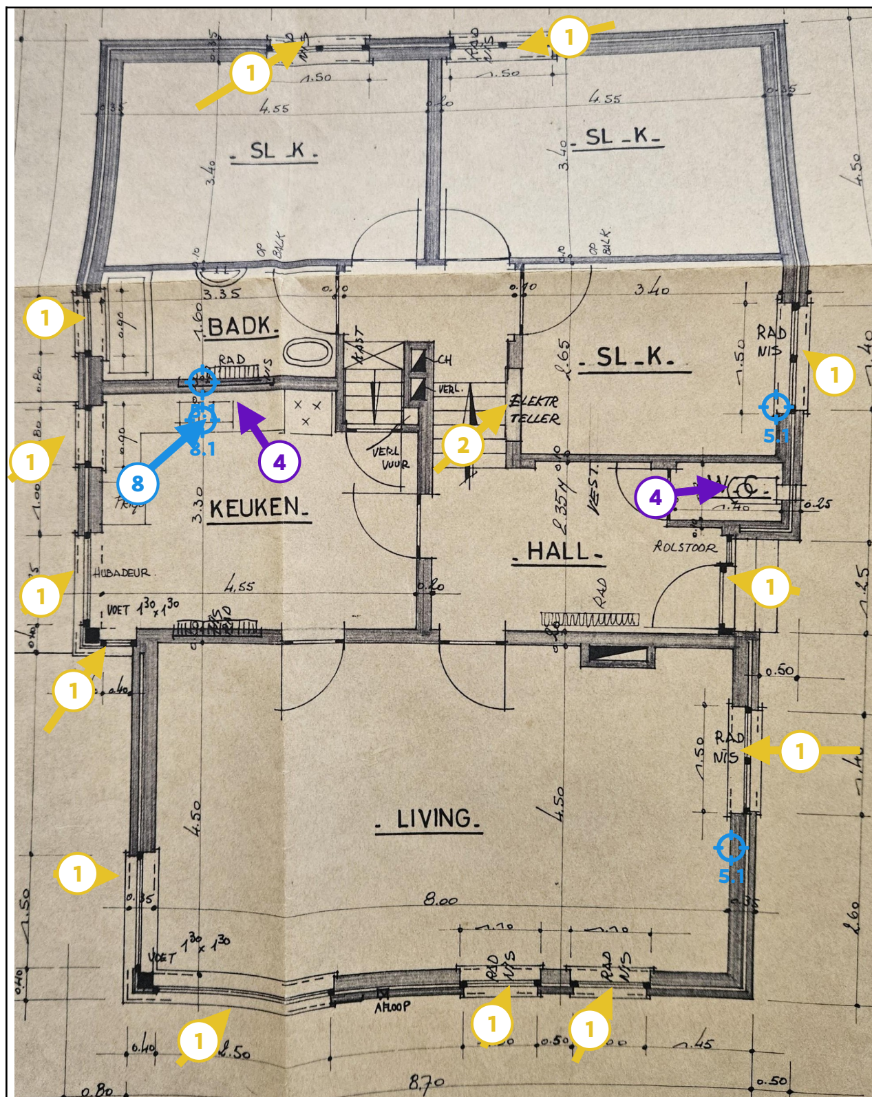
Legende van plan 1.2: gelijkvloers & 1e verdieping
