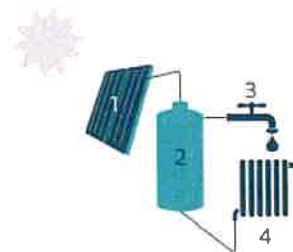
1. Zonnecollector | 2. Opslagvat zonneboiler | 3. Sanitair warm water | 4. Afghite-element voor ruimteverwarming (optioneel)
