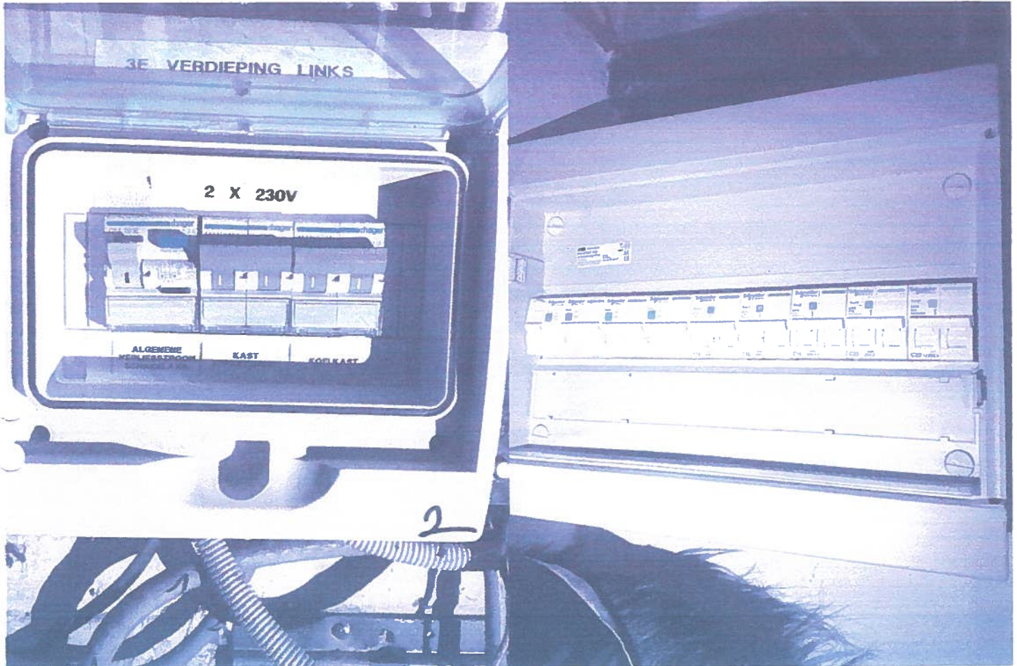
Verdeelbord 1
