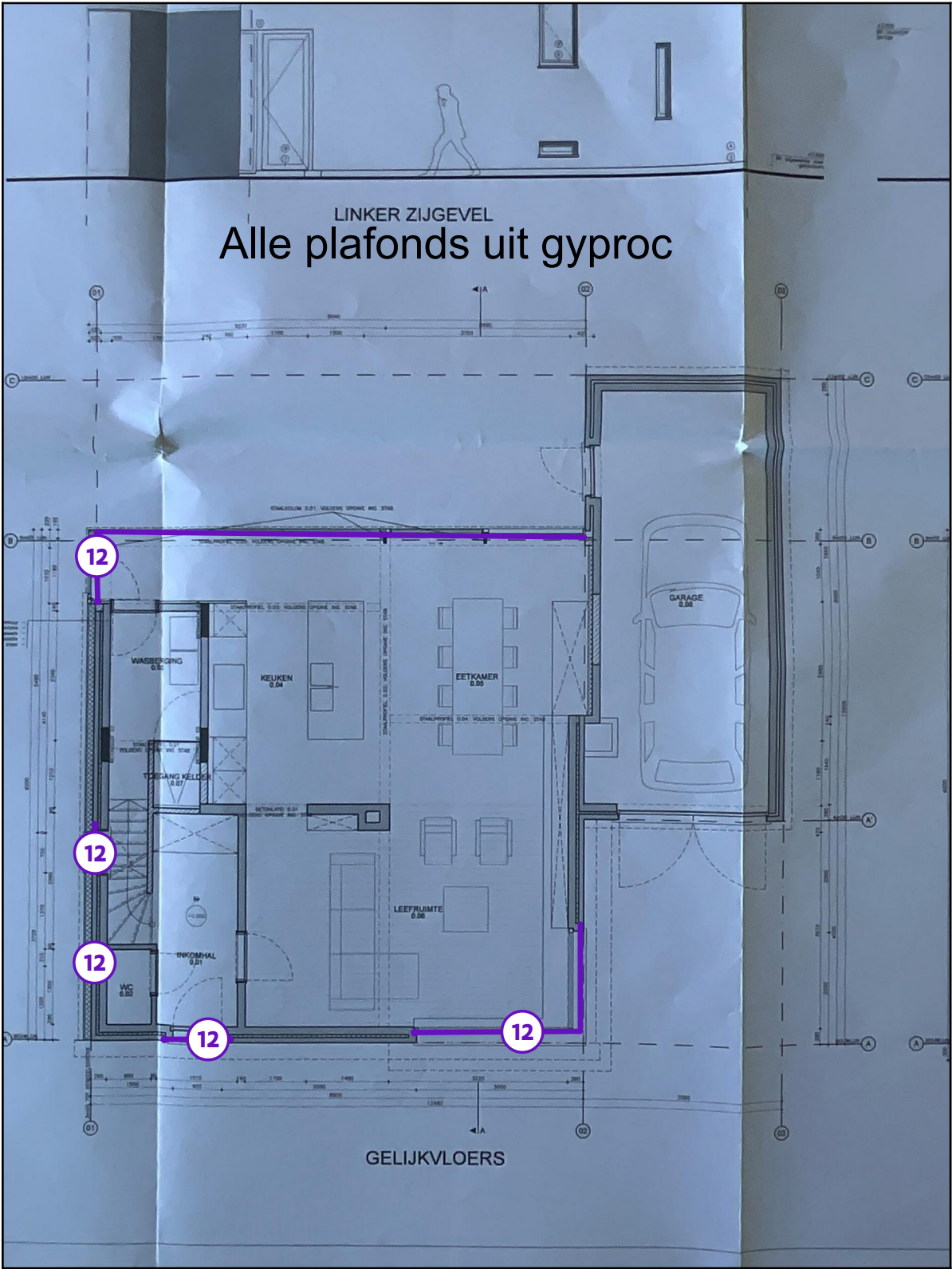
Legende van plan 1.5: Niveau 0 ramen
