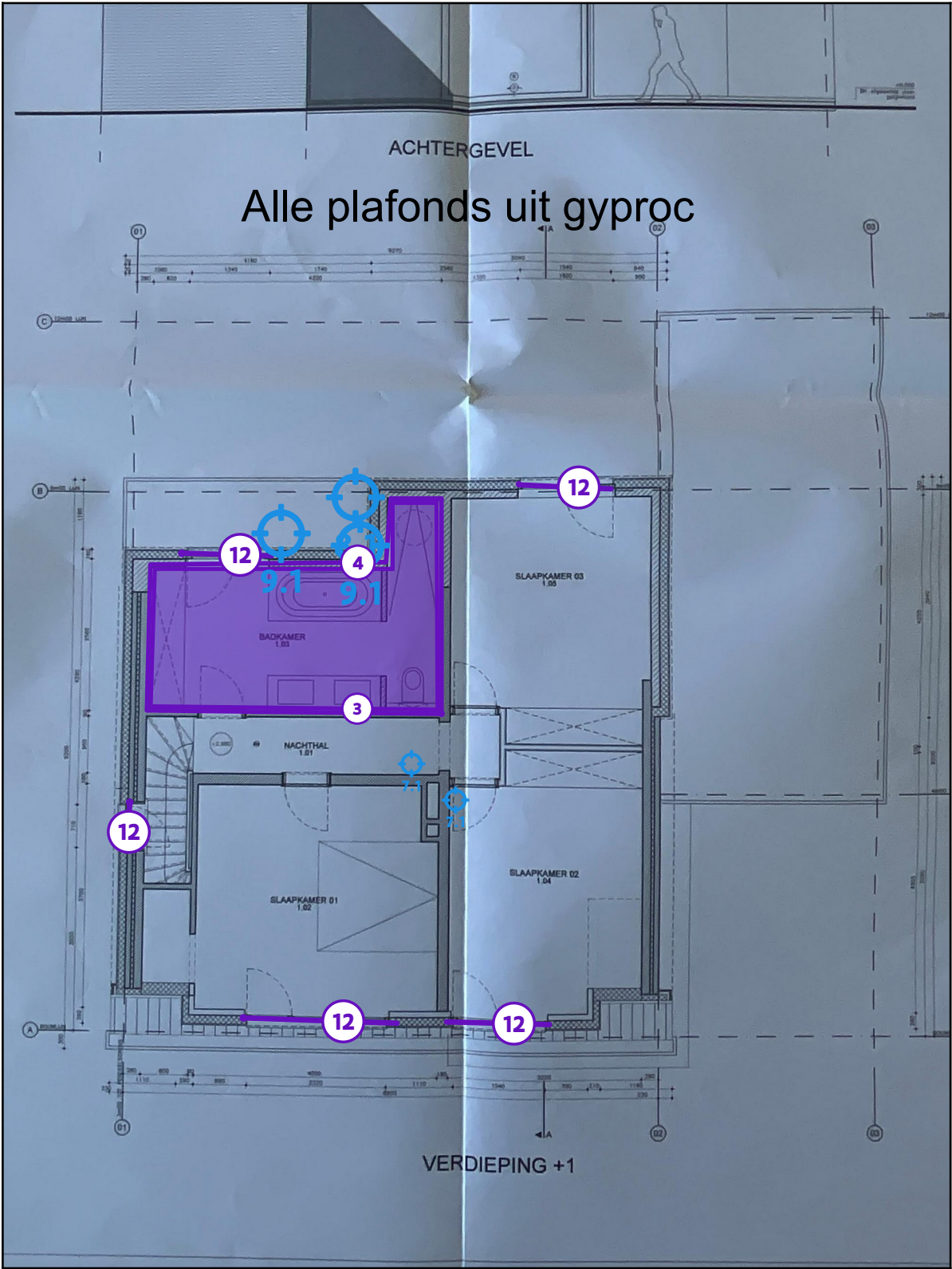
Legende van plan 1.3: Niveau +1
