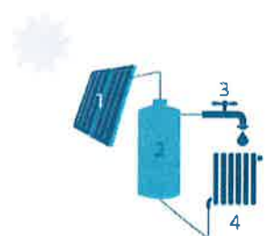
Zonnecollector (1), Opslagvat zonnecollector (2), Bad- en douchewater (3), Radiator (4)
