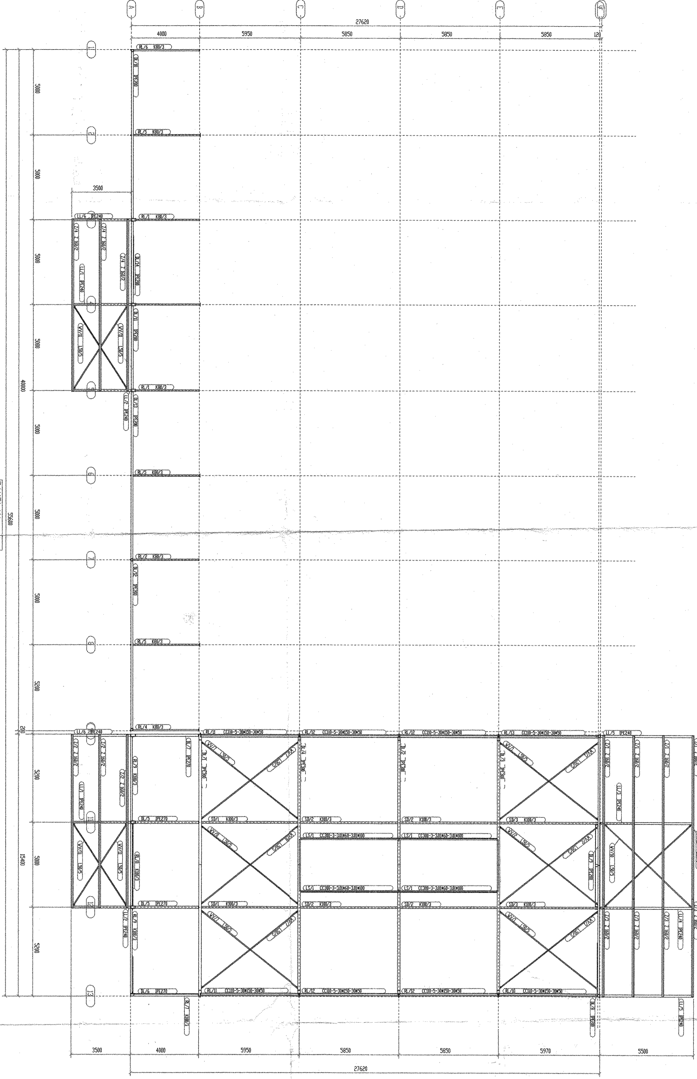
3D-STAHLGERÜST
