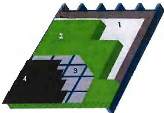
1. Damperschermb | 2. Isolatie | 3. Onderdak | 4. Dakbekleding
