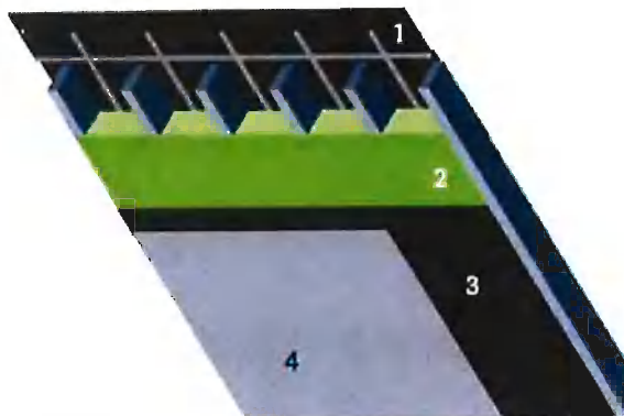
1. Onderdak | 2. Isolatie | 3. Damperschermb | 4. binnenafwerking
