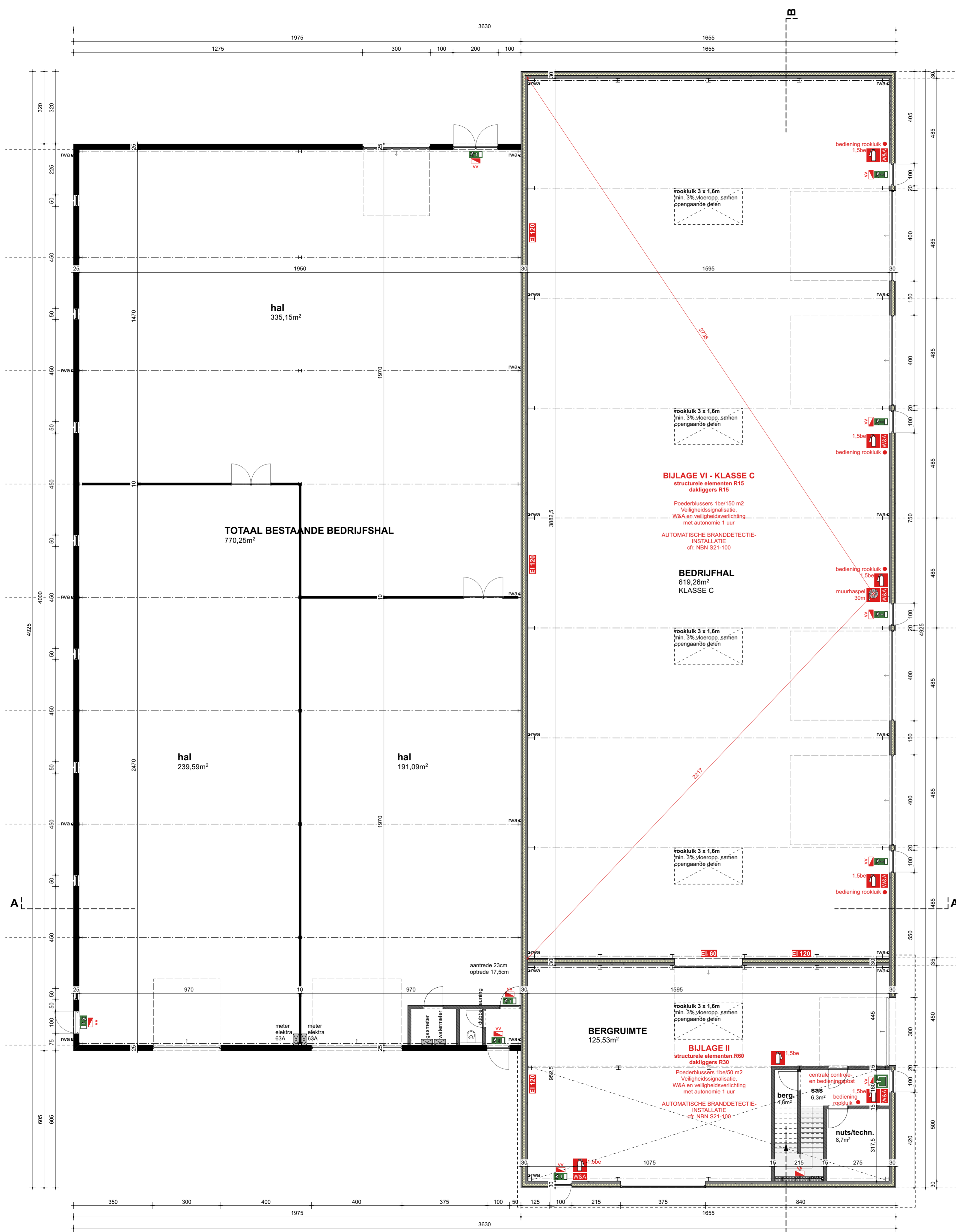
GELIJKVLOERS schaal 1/100
