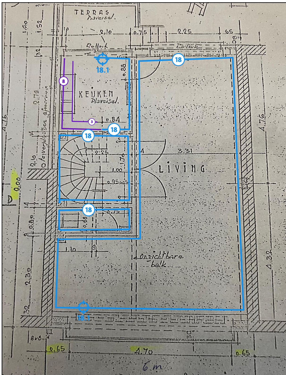
Legende van plan 1.3: Eerste verdieping
