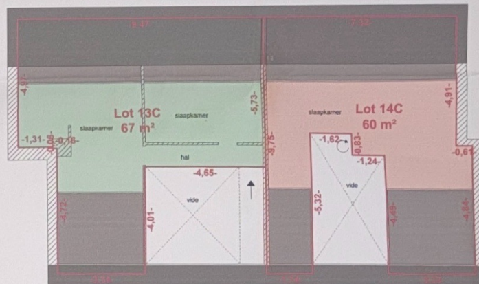
verdieping 3
