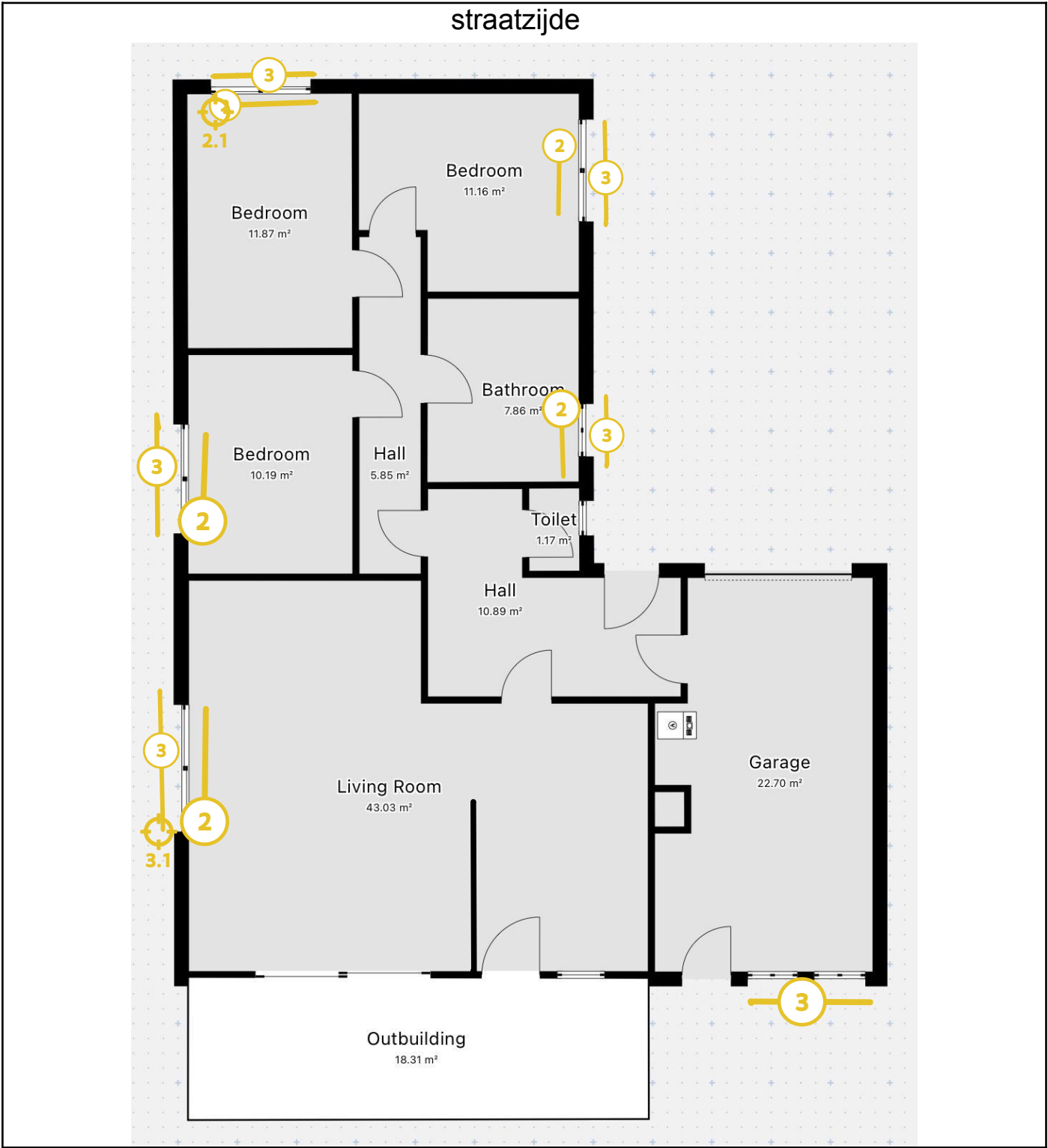
Legende van plan 1.2: Plan gelijkvloers woning
