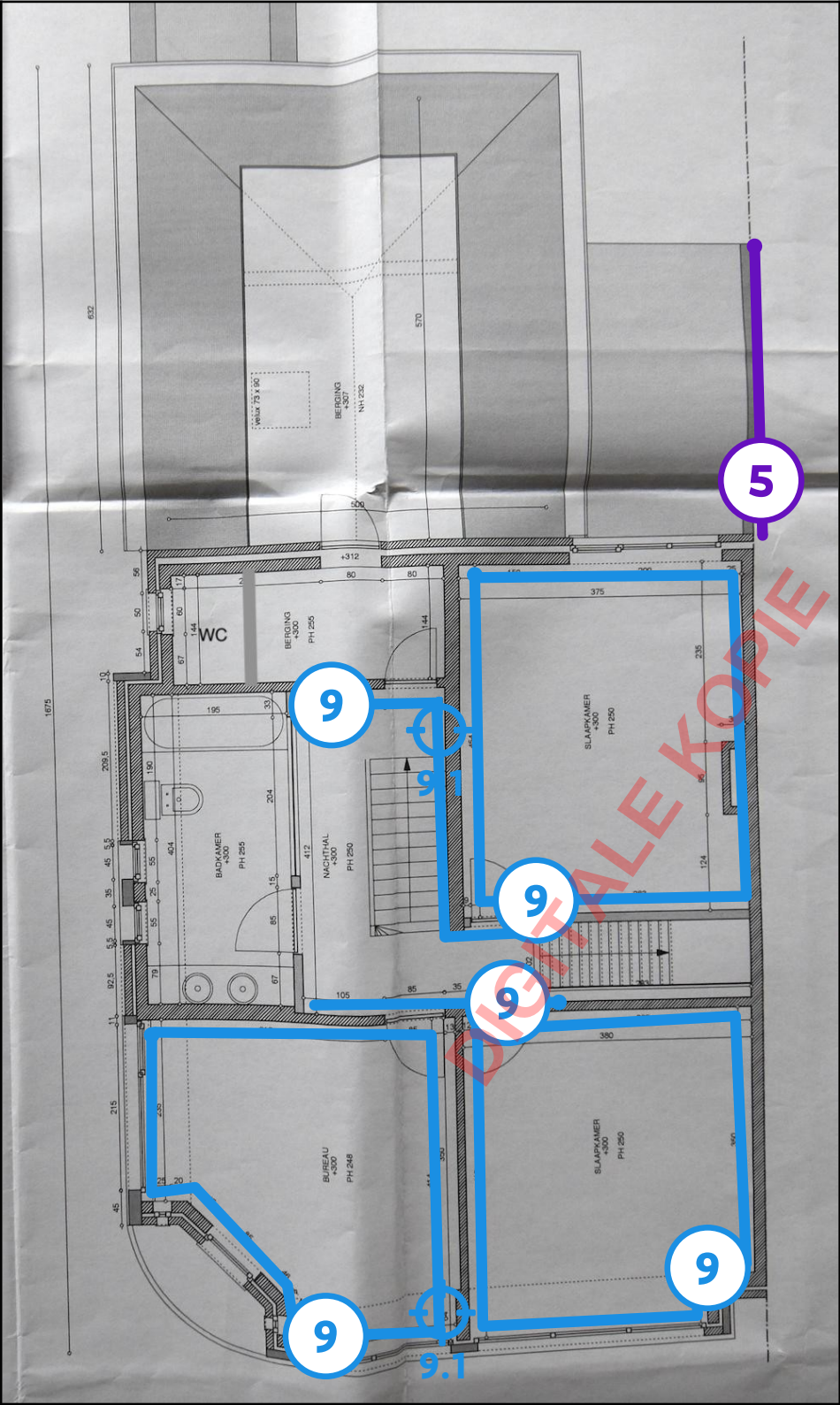
Legende van plan 1.3: Grondplan - 1ste verdieping
