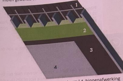
1. Onderdak | 2. Isolatie | 3. Dampscherm | 4. binnenafwerking
