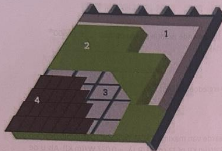
1. Dampscherm | 2. Isolatie | 3. Onderdak | 4. Dakbedekking
