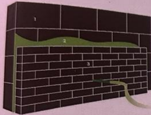
1. Dragende muur | 2. Ingeblazen isolatie | 3. Gevelsteen / gevelbekleding
