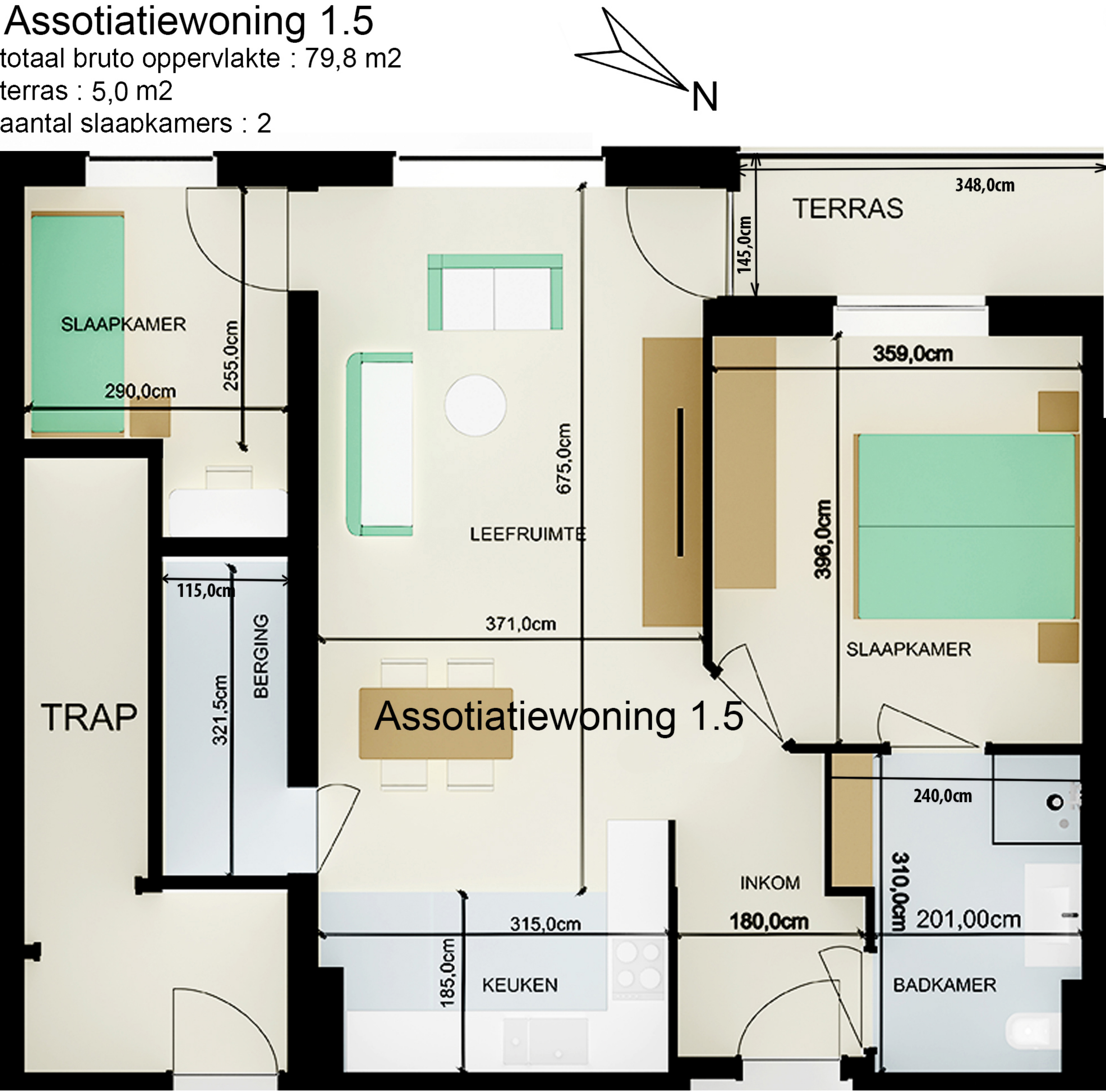
Wonen in Neeroeteren verdieping
