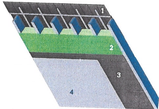
1. Onderdak | 2. Isolatie | 3. Dampscherm | 4. binnenafwerking
