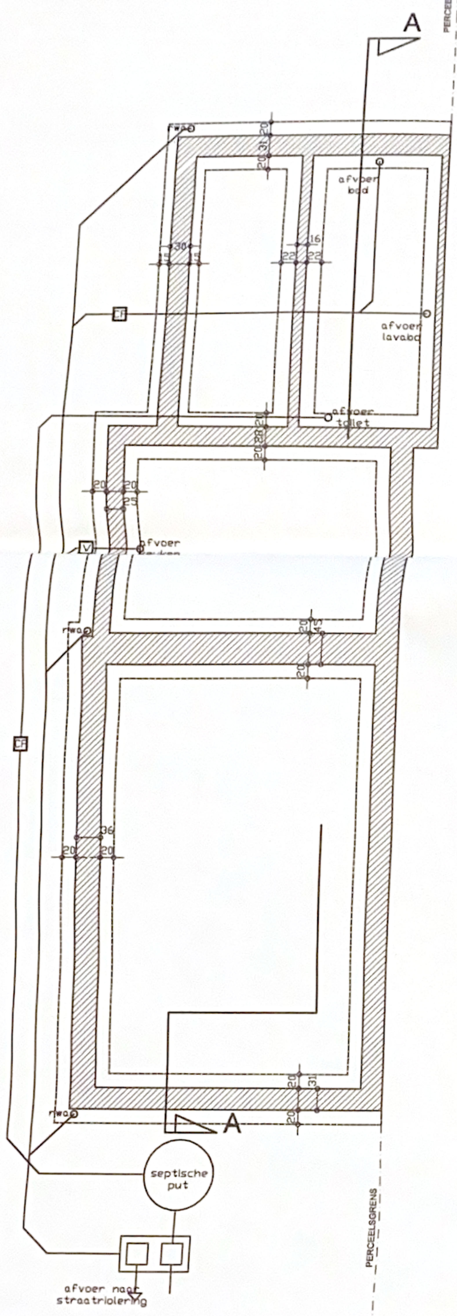
FUNDERINGS- & RIOLERINGSPLAN nieuwe toestand
