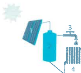
1 Zonnecollector | 2 Opslagvat zonnegedrukt H 2 O | 3 Sanitair warm water tap | 4 Aansluiting aan ruimteverwarming (radiator)
