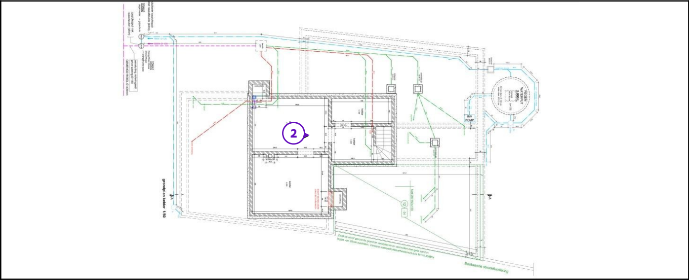
Legende van plan 1.1: Plan Kelder
