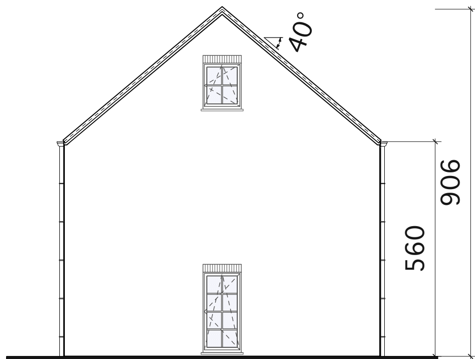
LINKER GEVEL
