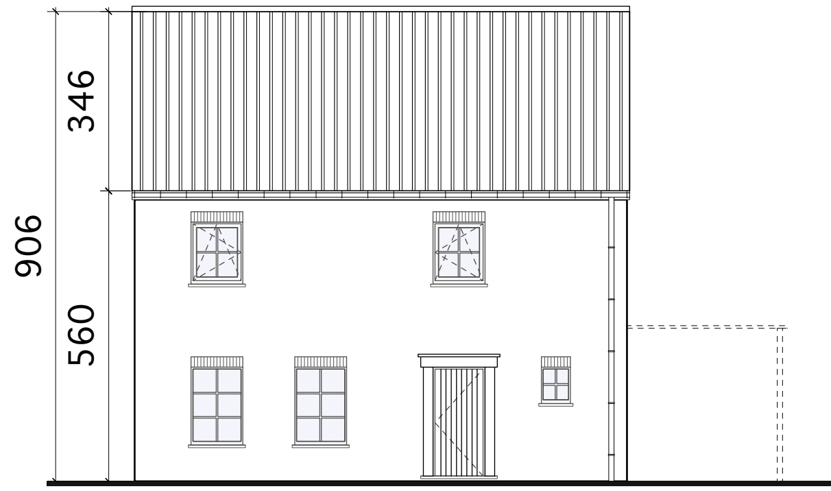
VOORGEVEL
