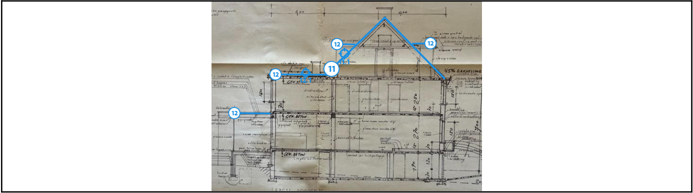
Legende van plan 1.11: Plan snede
