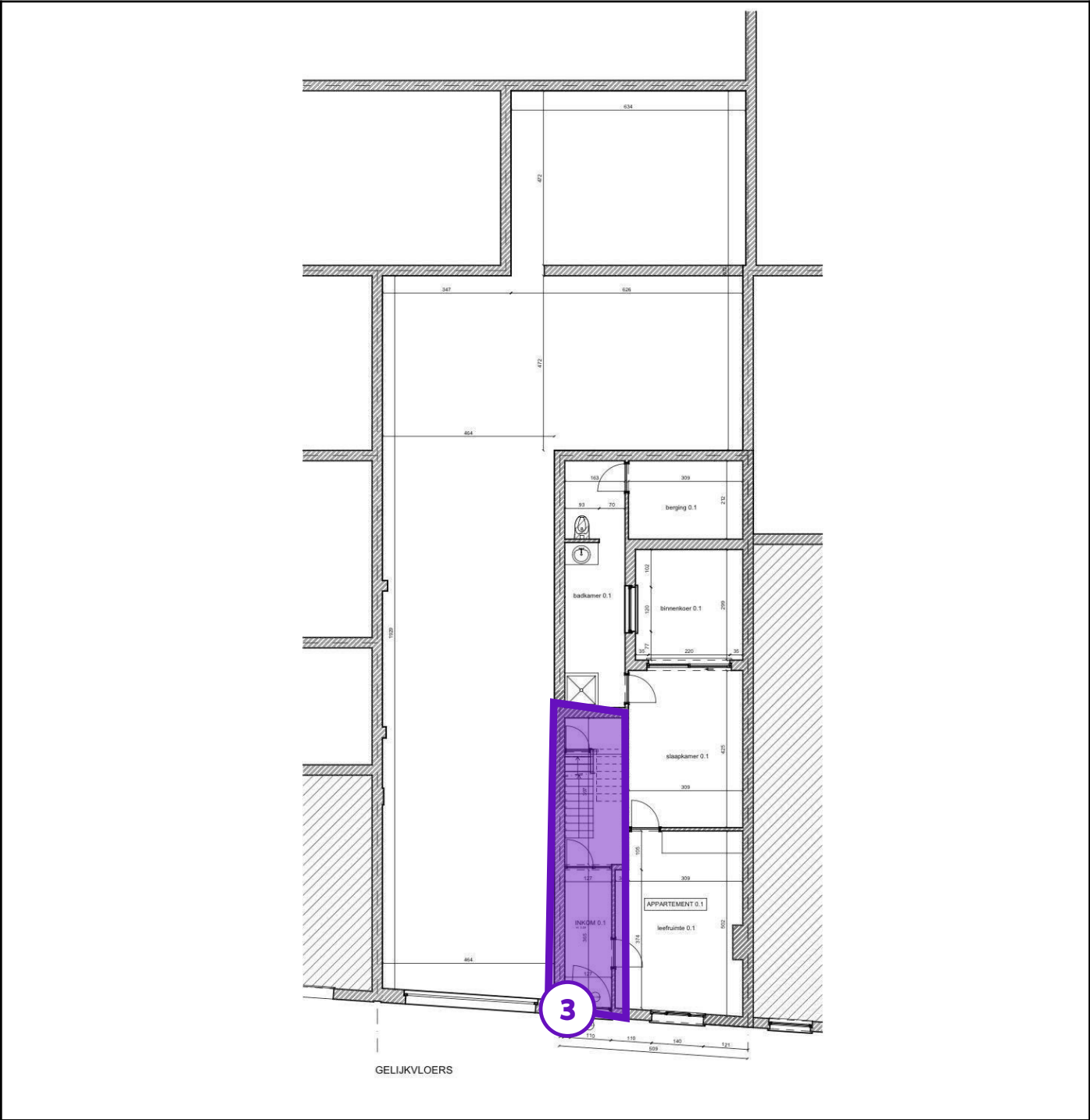
Legende van plan 1.6: GD - Gelijkvloers kopie kopie
