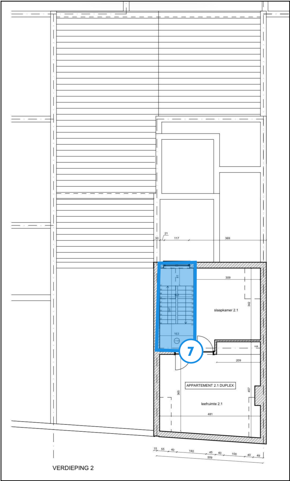
Legende van plan 1.11: GD - 2de Verdieping kopie
