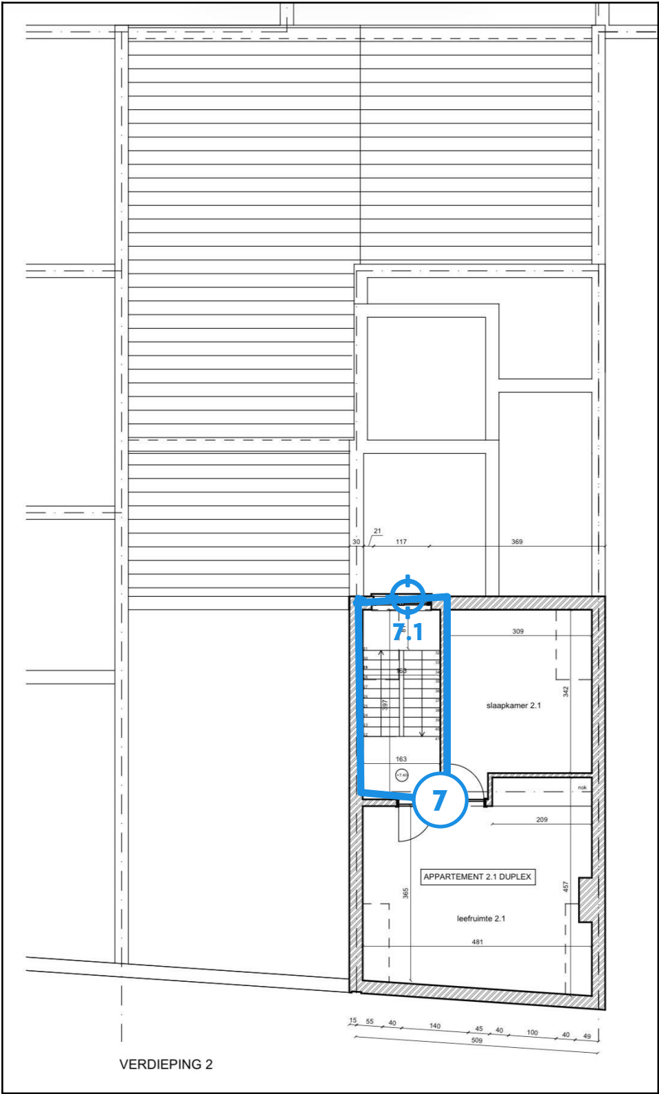
Legende van plan 1.10: GD - 2de Verdieping
