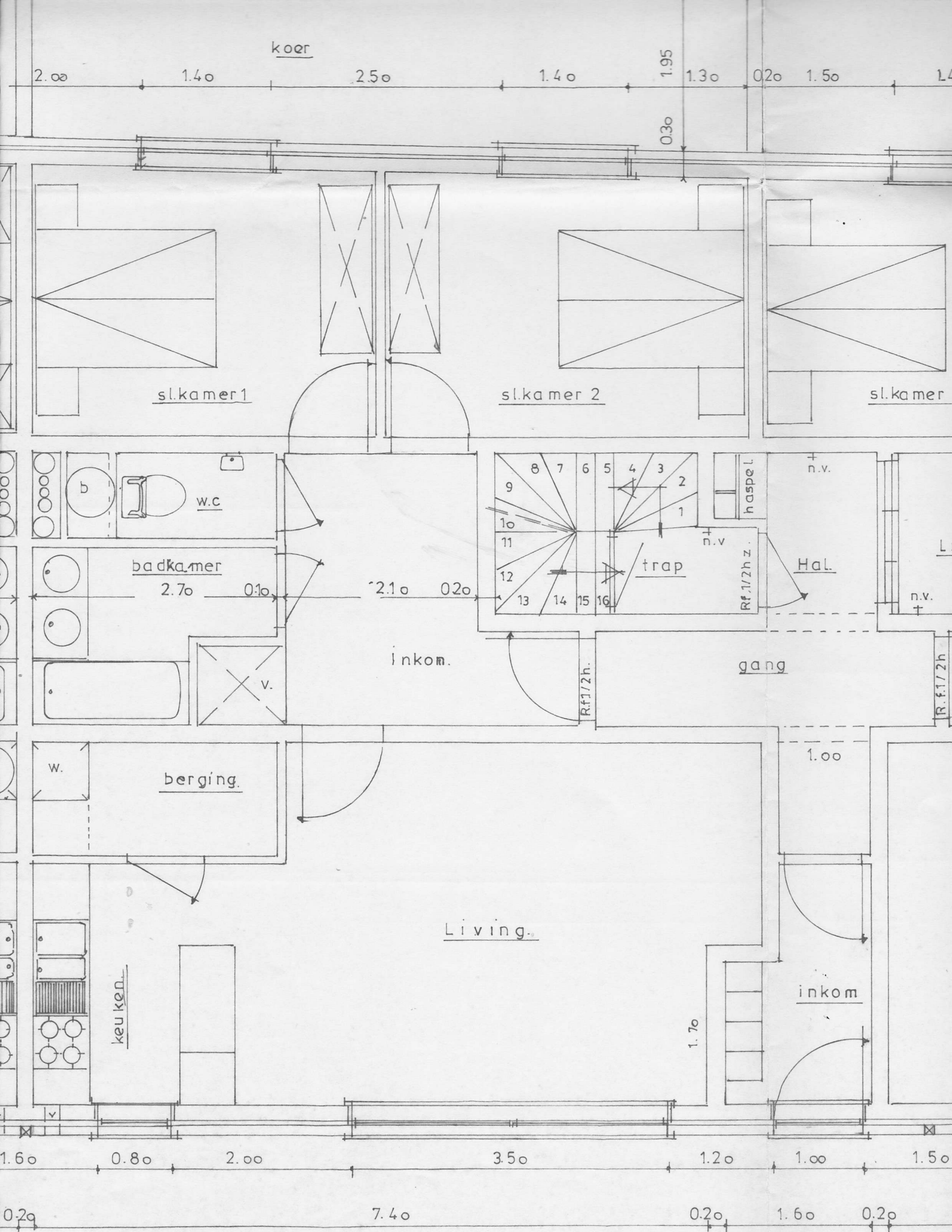
Plan: Gelijkvloers.
