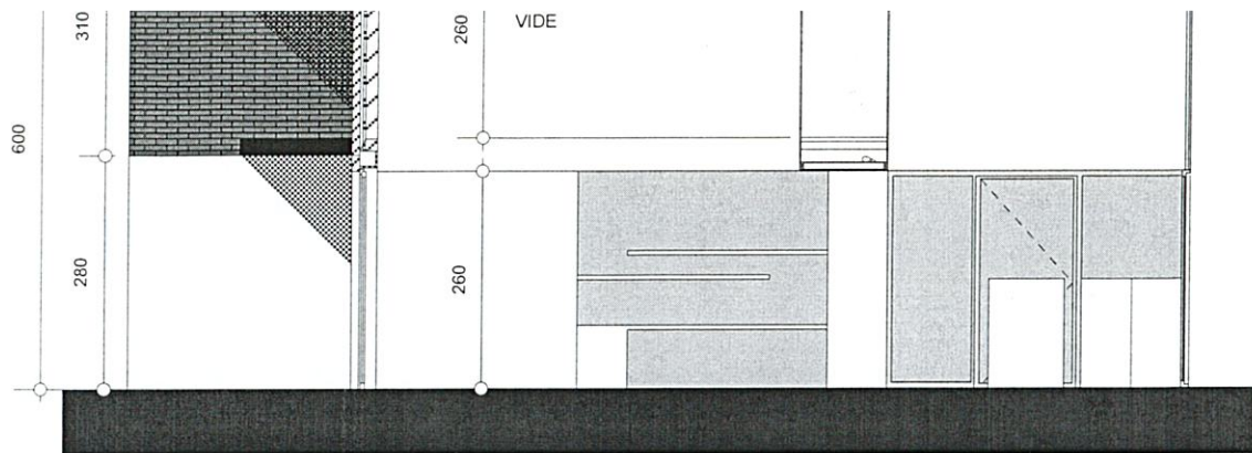
DOORSNEDE A-A
