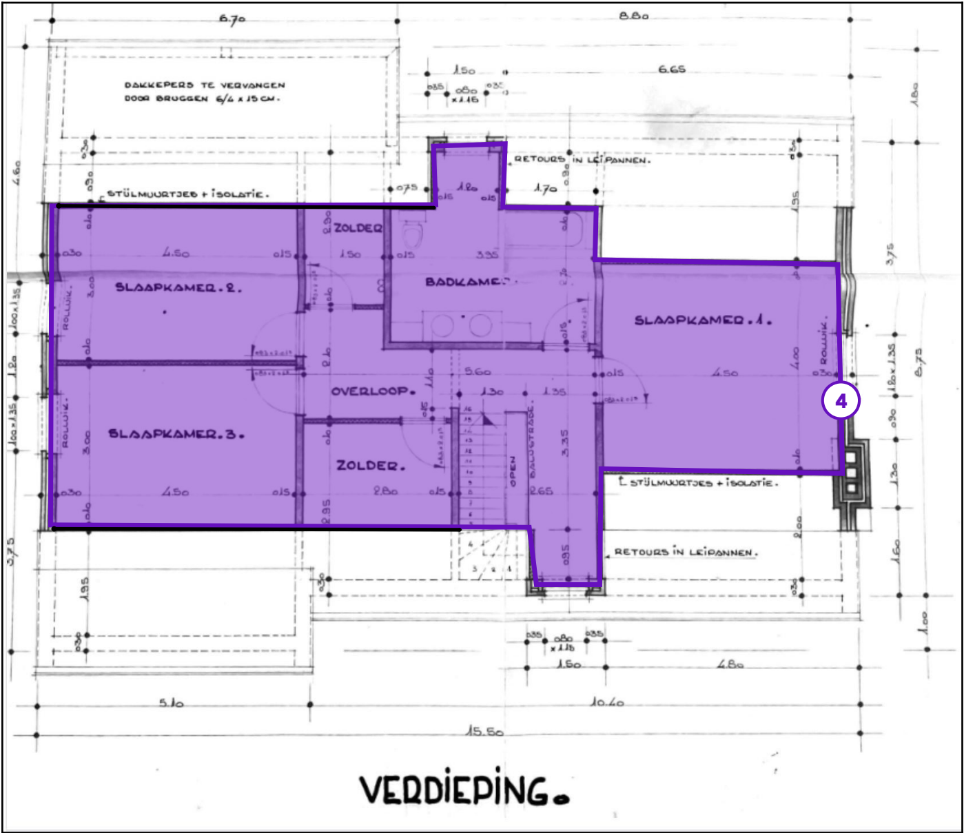
Legende van plan 1.9: V+1 : plafonds
