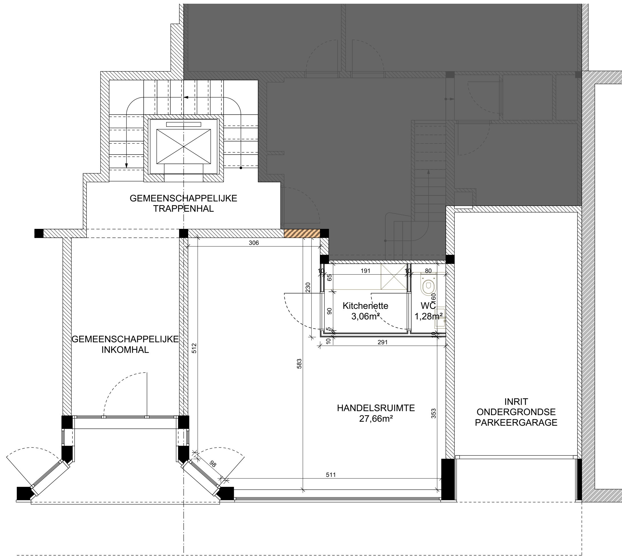
GRONDPLAN HANDELSRUIMTE - GELIJKVLOERS WEG naar AS 9, 3600 GENK
